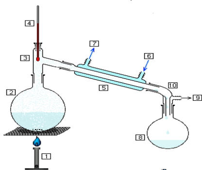
Destilační aparatura
